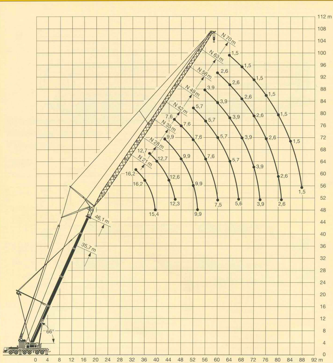
Teleskopausleger / Telescopic boom / Flèche télescopique: 66°
